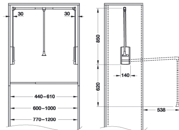
Einbau Mitte Schrankseitenwand
