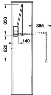
Einbau hintere Lochreihe
